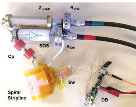
▲ Générateur SOS basé sur le transformateur d'impulsion saturable
