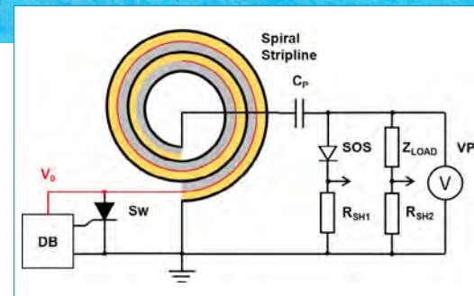
▲ Schéma électrique du générateur SOS basé sur une ligne de formation d'impulsions en spirale
