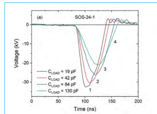
▲ Courbes de tension du générateur SOS sur une charge capacitive
